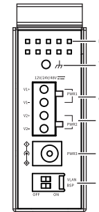
TL-SF1005工业级 上面板示意图
