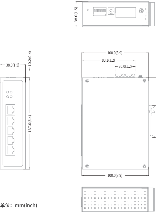
TL-SG1005工业级
