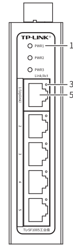
TL-SF1005工业级 前面板示意图
