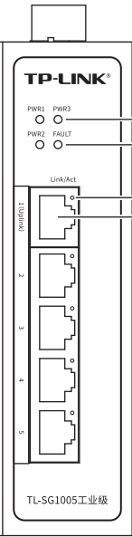
TL-SG1005工业级 前面板示意图
