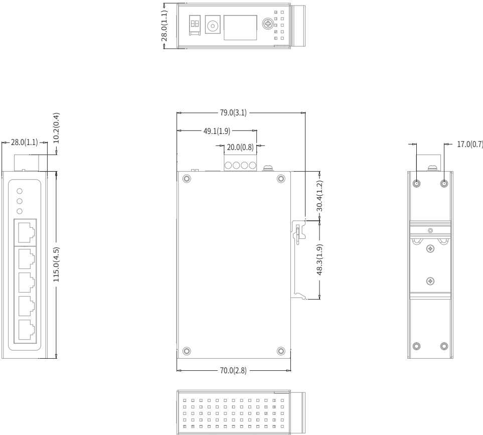
TL-SF1005工业级
